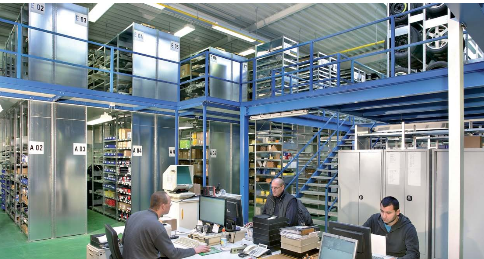
Das offen gestaltete Lager mit zweigeschossiger META CLIP® Anlage ist optimal auf die Kundenwünsche ausgerichtet, an den Serviceplätzen laufen alle Fäden zusammen
