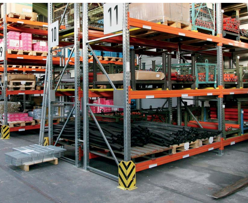
Dieses Lager umfaßt eine 2-geschossige, verzinkte META CLIP® Fachbodenregalanlage und eine META MULTIPAL® Palettenregalanlage
