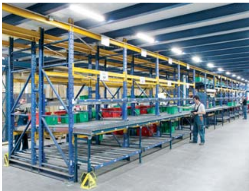
META Kommissionierregal mit einer zusätzlichen, querlaufenden Transport-Rollenbahn zur Beschickung der Regale.
